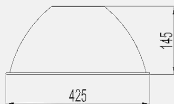
Chóa đèn 60°
