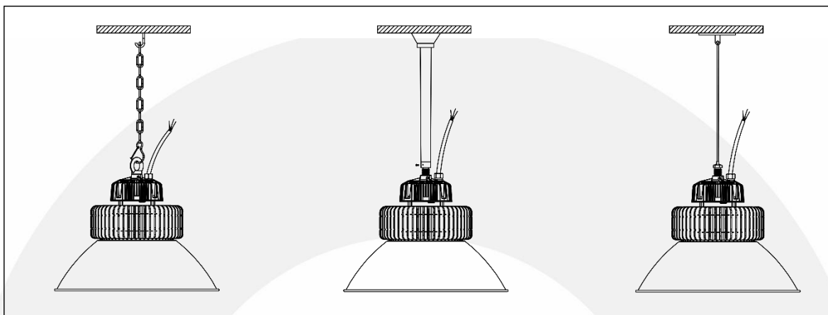
DÒNG XÍCH
